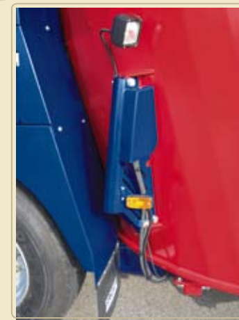
Противорезающие пластины с гидроприводом регулируются прямо из кабины машины.
